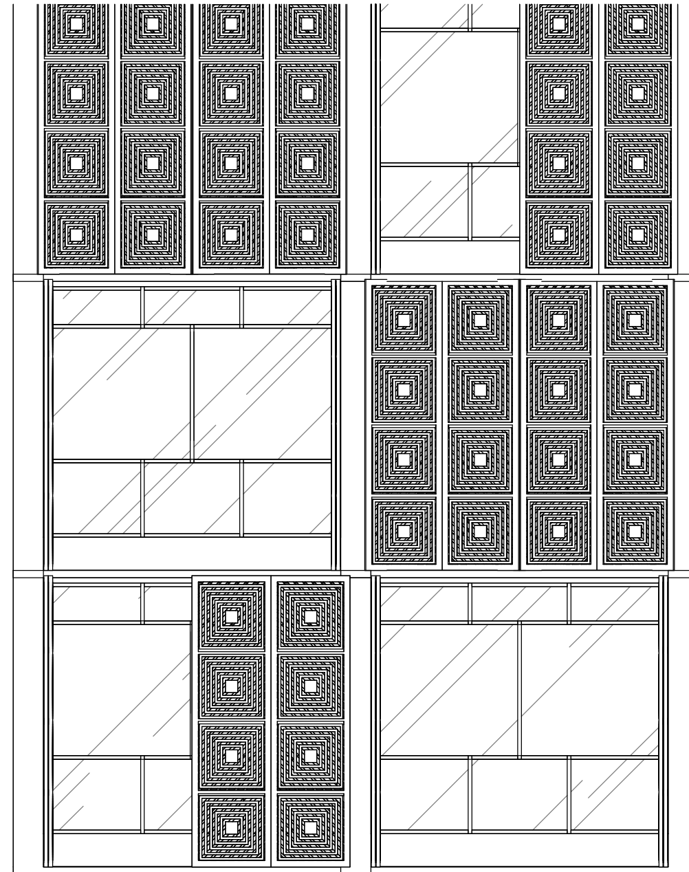
2 ELEVAÇÃO 1 : 50
