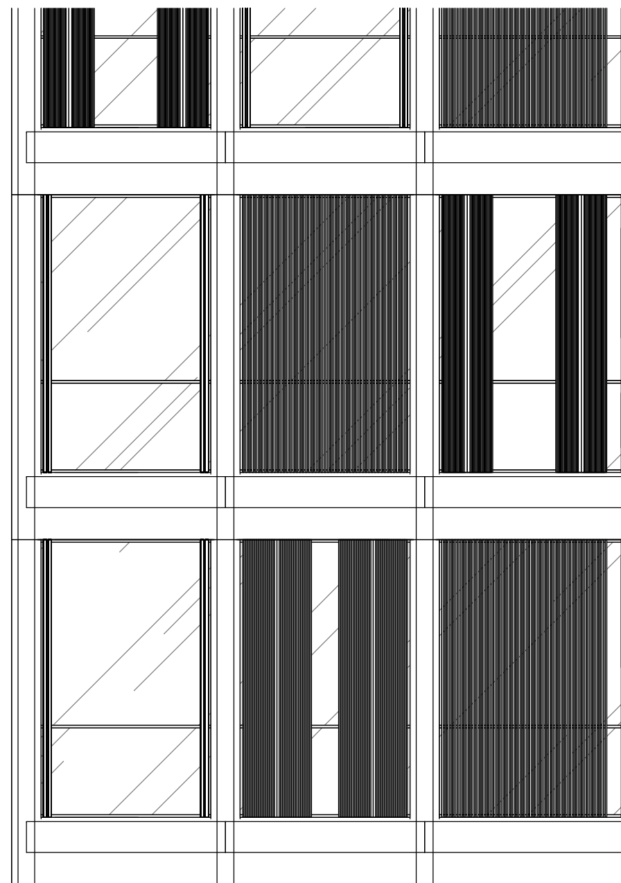
2 ELEVAÇÃO 1 : 50
